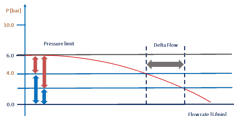
Fig. 56: Graphique de la pression du système
