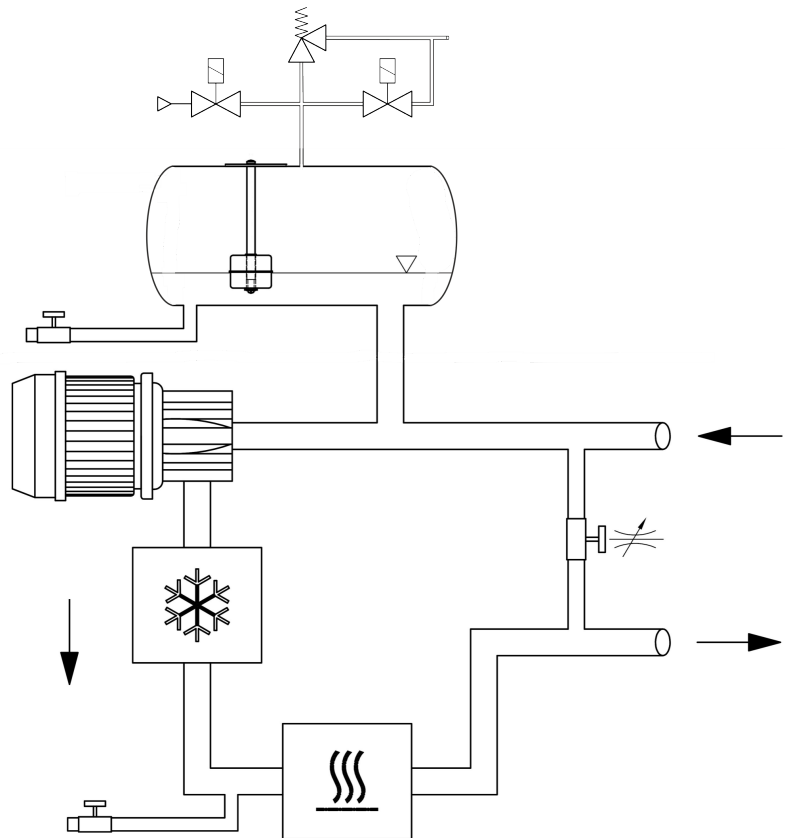
Fig. 9: Schéma du circuit hydraulique des appareils IN P
