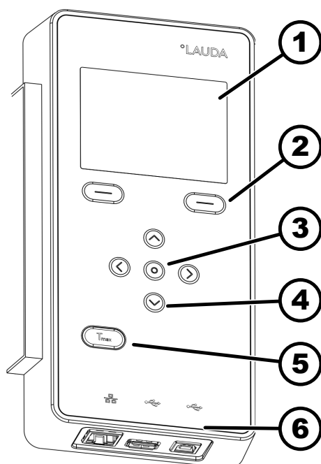
Fig. 28: Unité de commande
