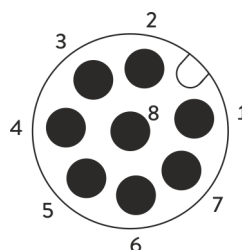
Fig. 12: Affectation des broches de l'interface de sécurité
