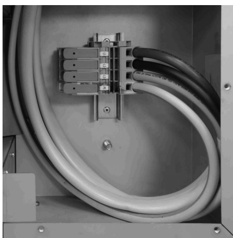
Fig. 22: Bornes présentes dans le boîtier de raccordement
