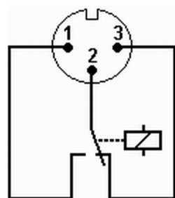
Fig. 15: Connecteur à bride (en façade) à l'état de panne
