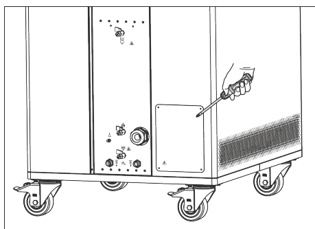
Fig. 20: Panneau de revêtement devant le boîtier de raccordement
