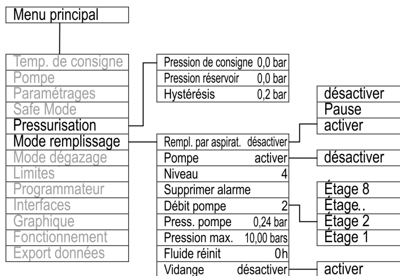
Fig. 40: Structure de menus de la pressurisation
