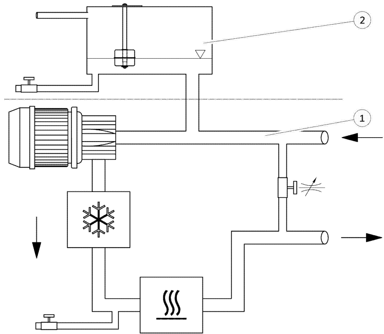
Fig. 8: Schéma du circuit hydraulique des appareils IN XT
