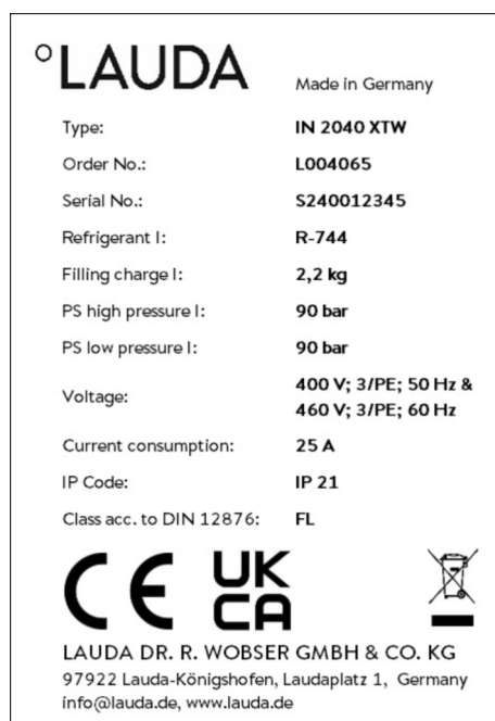
Fig. 10: Plaque signalétique (exemple)
